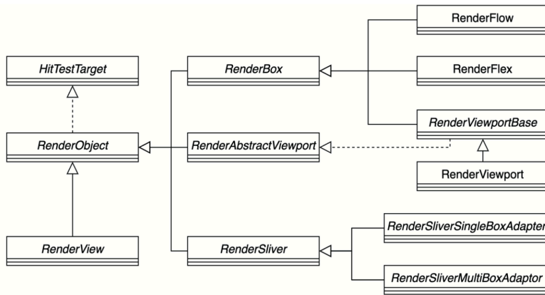
图 5-3 RenderObject 关键类及其子类
